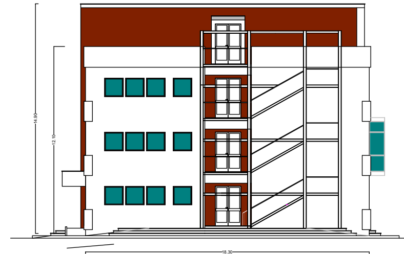
PROSPETTO LATO NORD
