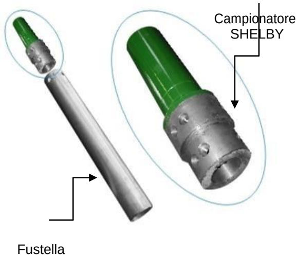
Foto 10: Campionatore a pareti sottili impiegato per il prelievo di campioni indisturbati.
