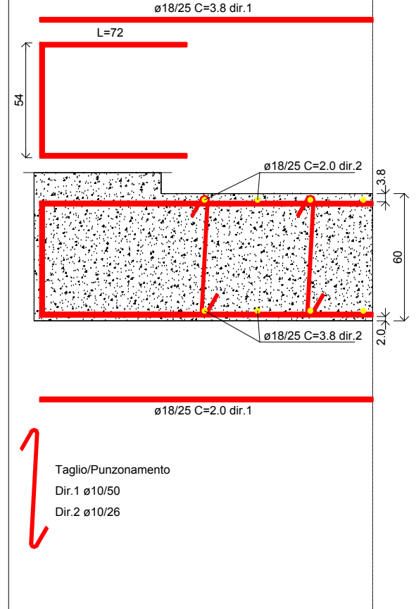
Particolare armatura (scala 1:20)
