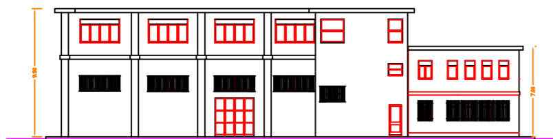
Prospetto Est
