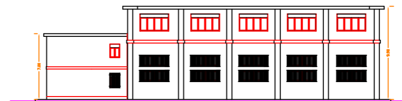
Prospetto Ovest
