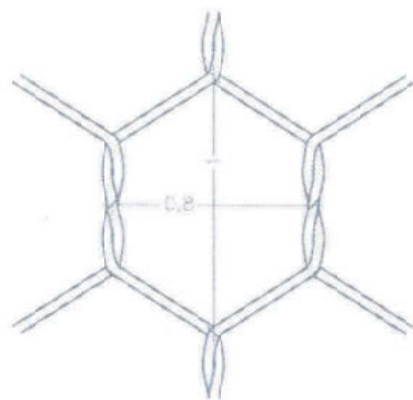
DETTAGLIO N° 1
