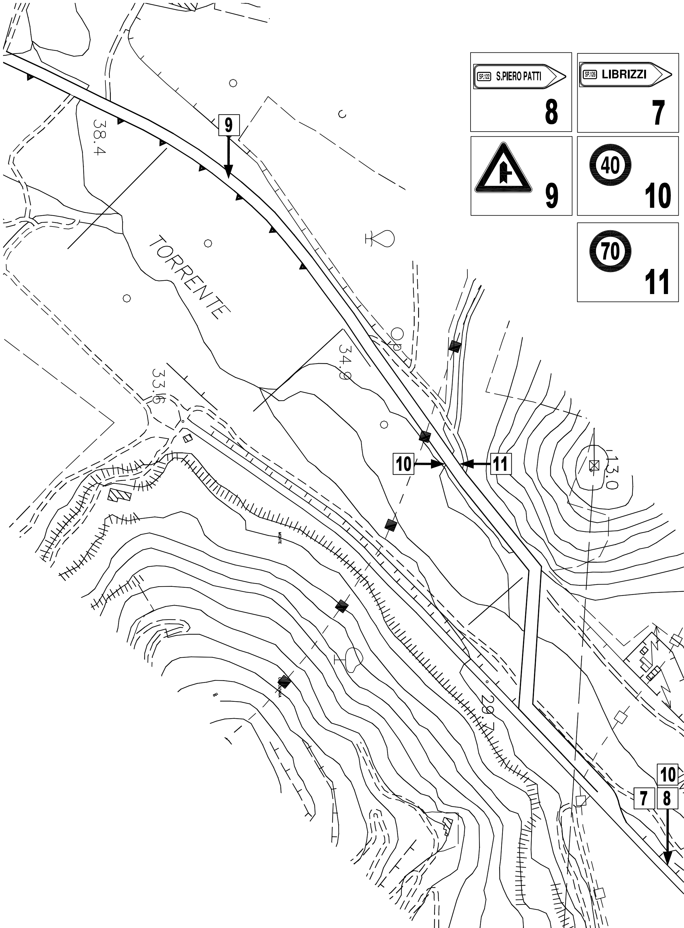
TAV. 4 2° LOTTO - SEGNALETICA VERTICALE POSIZIONAMENTO DA Km 0+00 A Km 1+00 SCALA 1: 2.500
