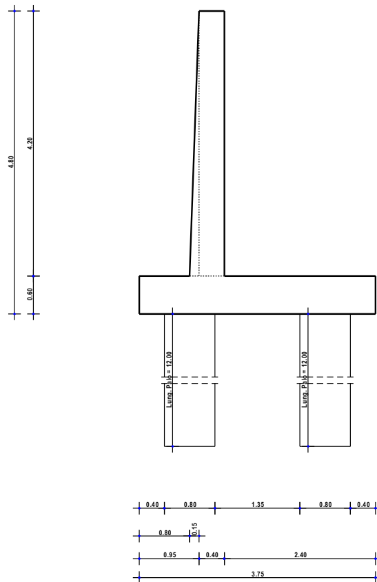
Sezione 1 - Vista Sezione
