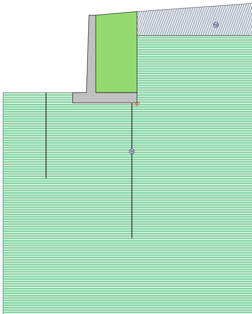
SEZIONE 1 - STRATI
