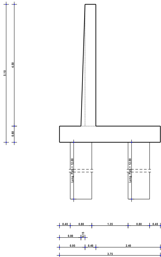
Sezione 1 - Vista Sezione
