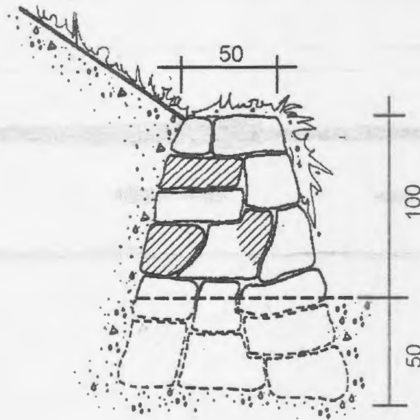
Prospetto - Sezione laterale
