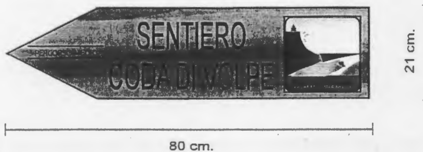
Schema di montaggio
